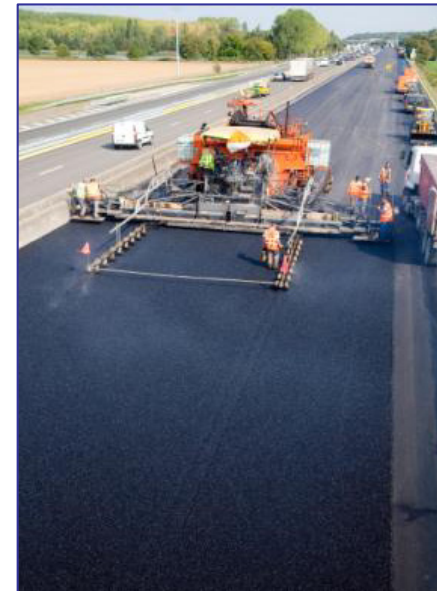
Autoroute A26 en Champagne
